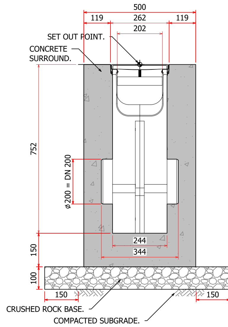
HAURATON RECYFIX PRO 200 TRASHBOX
