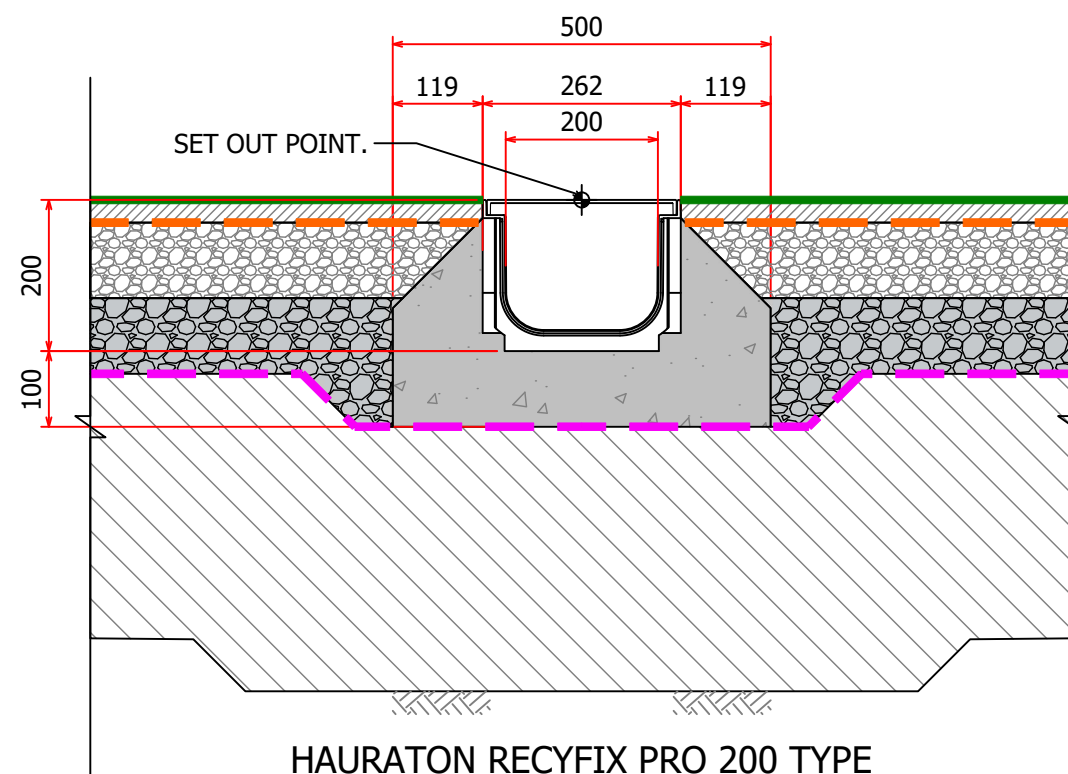
HAURATON RECYFIX PRO 200 TYPE 010 TRENCH
