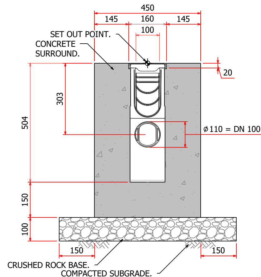
HAURATON RECYFIX PRO 100 TRASHBOX
