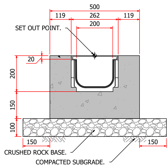
HAURATON RECYFIX PRO 200 TYPE 10 TRENCH
